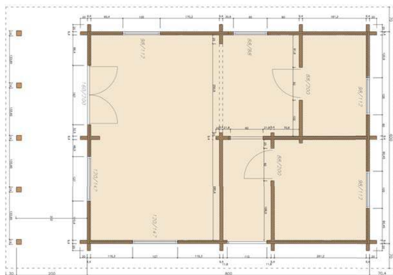
GRUNDRISS EG
