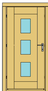
T28-ET-3 Madriers de: 28 mm masse: 84 x 184 cm
