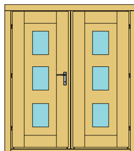
T28-DT-3 Madriers de: 28 mm masse: 150 x 184 cm
