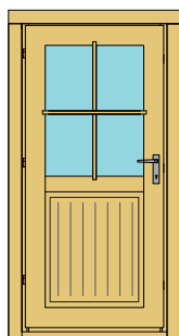
T28-ET Madriers de: 28mm masse: 84 x 184 cm
