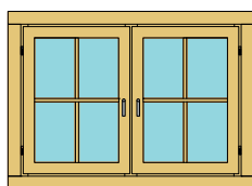
F28-DF Madriers de: 28 mm masse: 110 x 92 cm
