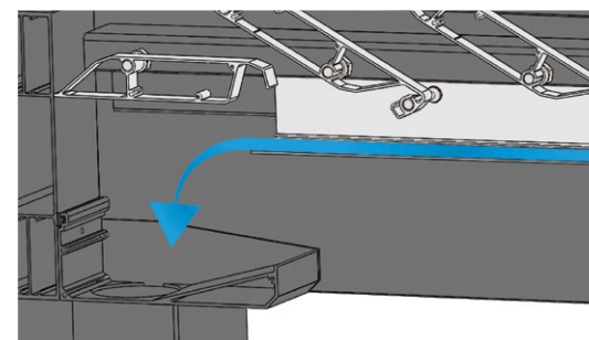
Évacuation des eaux
