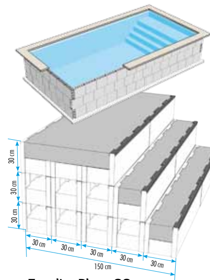
Escalier Plage 90 cm : Largeur du bassin.
