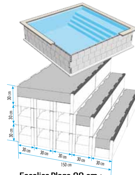
Escalier Plage 90 cm : Largeur du bassin.
