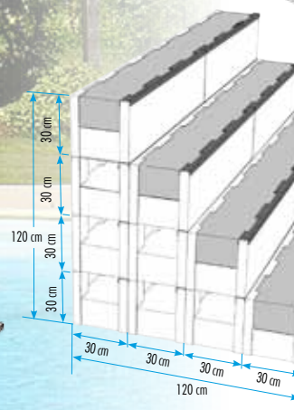
Escalier standard : Largeur du bassin.
