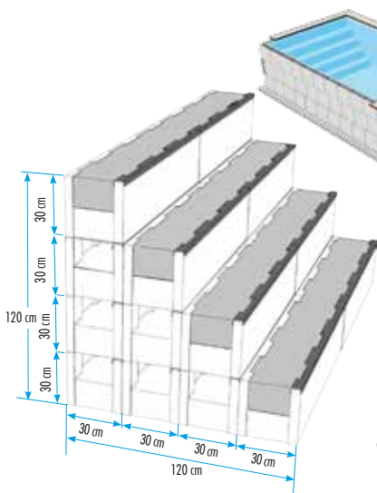
Escalier standard : Largeur du bassin.
