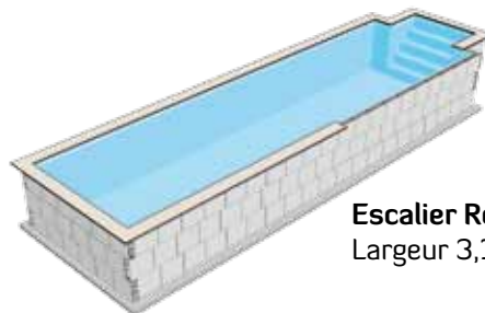
Escalier Roman extérieur : Largeur 2,77 m.
